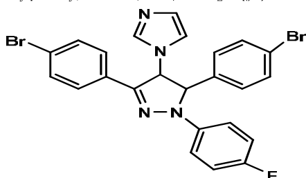
Fig.38. 3,5-bis(4-bromophenyl)-1-(4-fluorophenyl)-4-(1 H -imidazol-1-yl)-2-pyrazoline
