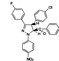
Fig.27. 4-(4-chlorophenyl)-3-(4-fluorophenyl)-1-(4-nitrophenyl)-2-pyrazolin-5-yl(phenyl)methanone
