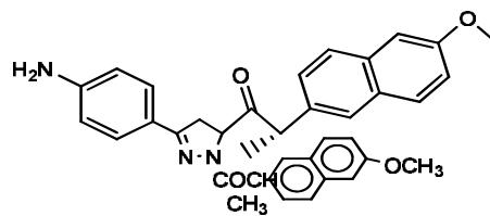
Fig.29. 1-(3-(4-aminophenyl)-1-(2-(6-methoxynaphthalen-2-yl)propanoyl)-2-(6-methoxynaphthalen-2-yl)propan-1-one
