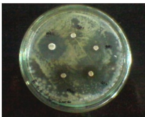
B. subtilis
