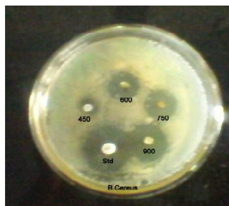
B. cereus
