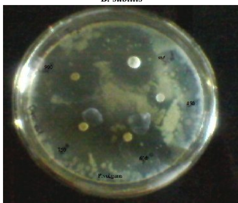
P. vulgaris
