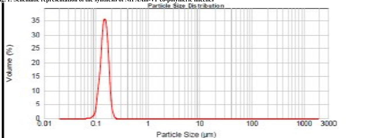
Fig. 2: Micellar size
