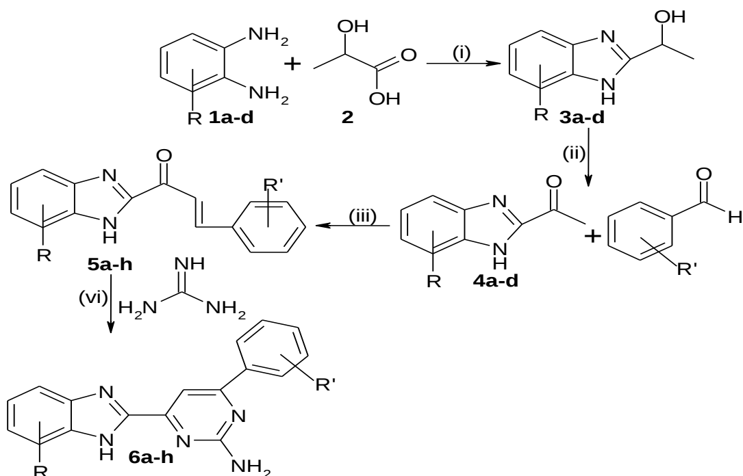
Scheme 1 (i) HCl, reflux, 22-24 h, (ii) K_2Cr_2O_7 , H_2SO_4 , 2-3 h, (iii) EtOH, 60% KOH, 4-5 h, (iv) AcOH, reflux, 4-5 h. 1/3/4a-d R = a) H, b) 4-CH 3 , c) 4-Cl; d) 4-NO 2 . 5/6 a-h R = a) H, b) H, c) H, d) 4-CH 3 , e) 4-CH 3 , f) 4-Cl, g) 4-Cl, h) 4-NO 2 . 5/6 a-h R' = a) H, b) 4-OCH 3 , c) 3,4-OCH 3 , d) H, e) 4-C 2 H 5 , f) 4-C 2 H 5 , g) 4-NO 2 , h) 4-C 2 H 5 .
